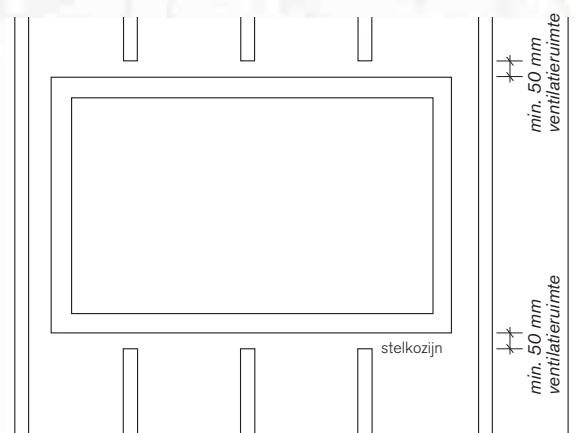
Kozijnen in chaletbouw
